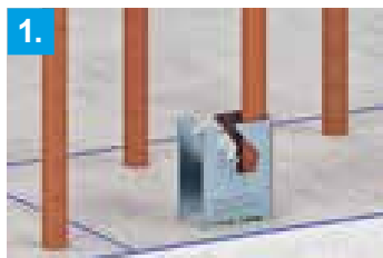
1. Manschette um das Anschluss-eisen legen
