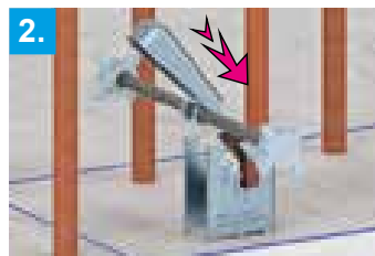
2. Der Keil gleitet automatisch in die richtige Halterung
