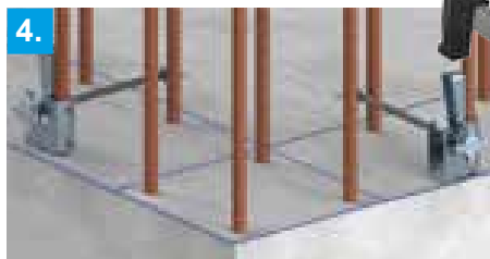
4. Fixierung mit einem Hammerschlag
